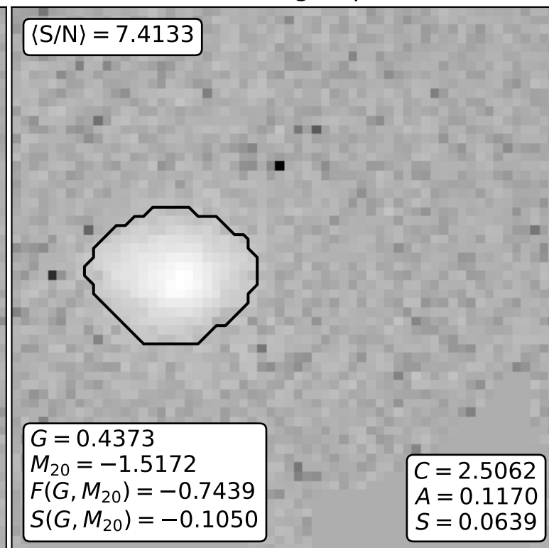
Gini Segmap
