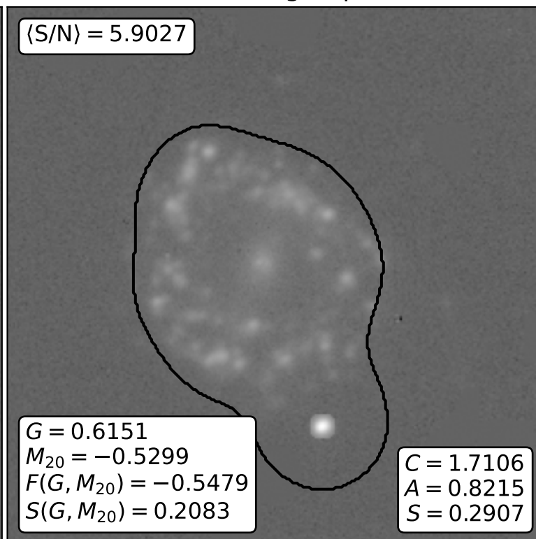
Gini Segmap
