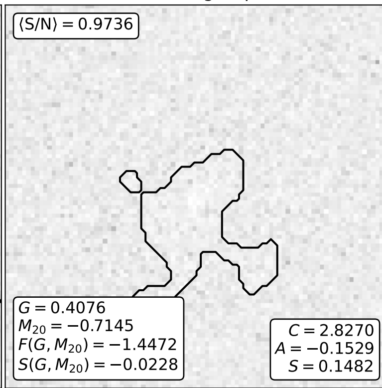
Gini Segmap
