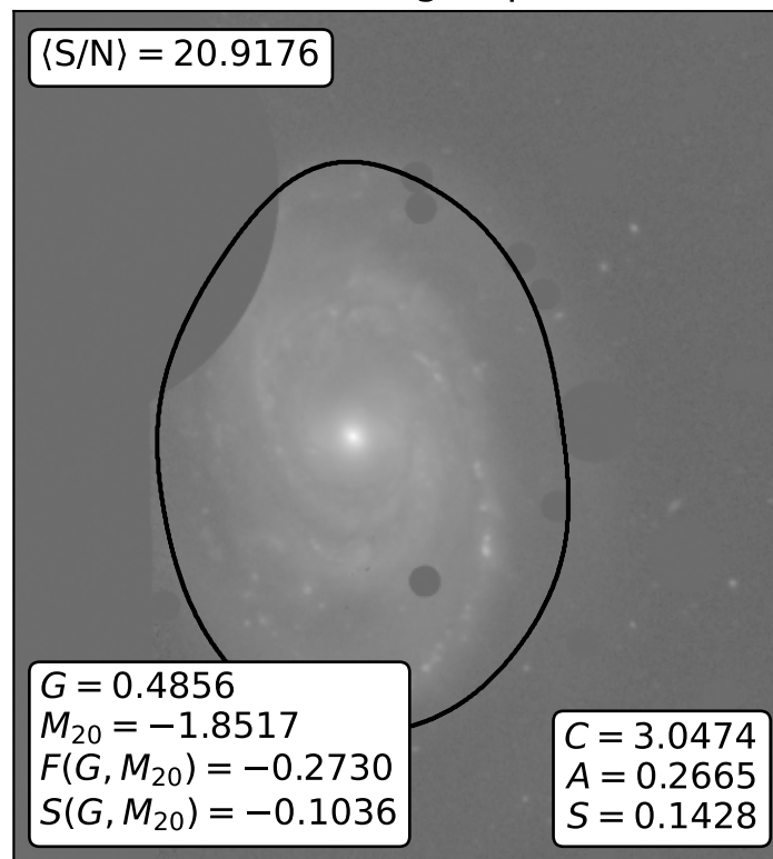
Gini Segmap
